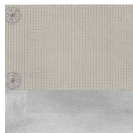
Aquapanel – preparation for cladding Aquapanel – Vorbereitung zum Fliesenlegen Aquapanel – préparation du lambris 🔗
